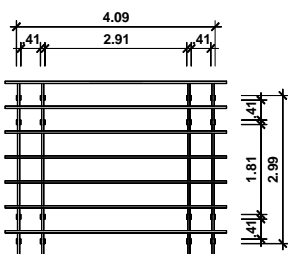
Abbildung: Grundriss Art.-Nr. 7110
