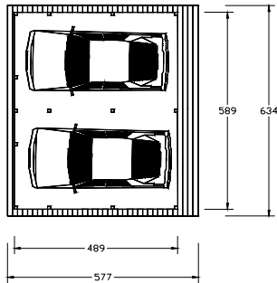
Draufsicht Art.-Nr. 4208
